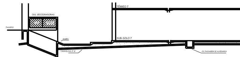
CORTE A-A
